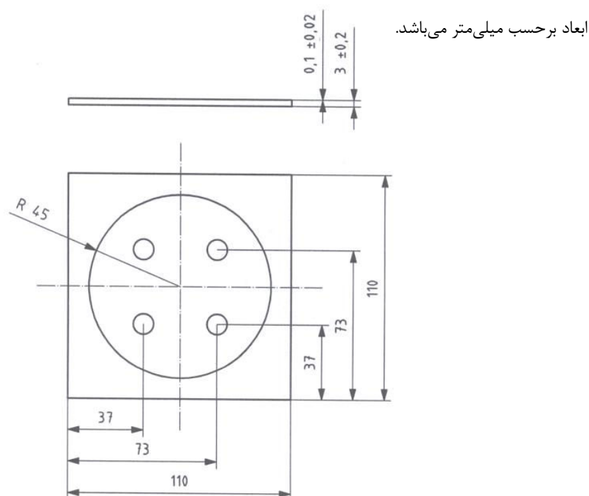
شکل ۲ - صفحه حایل
