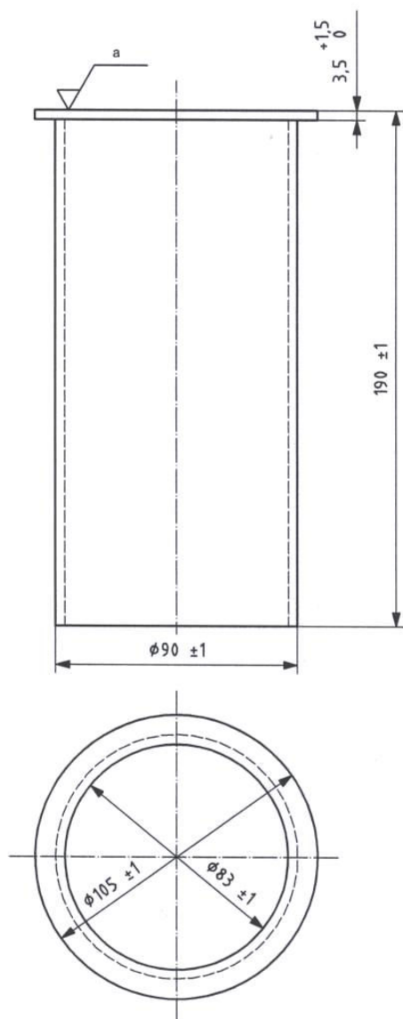
شکل ۱ - بشر شیشه‌ای
