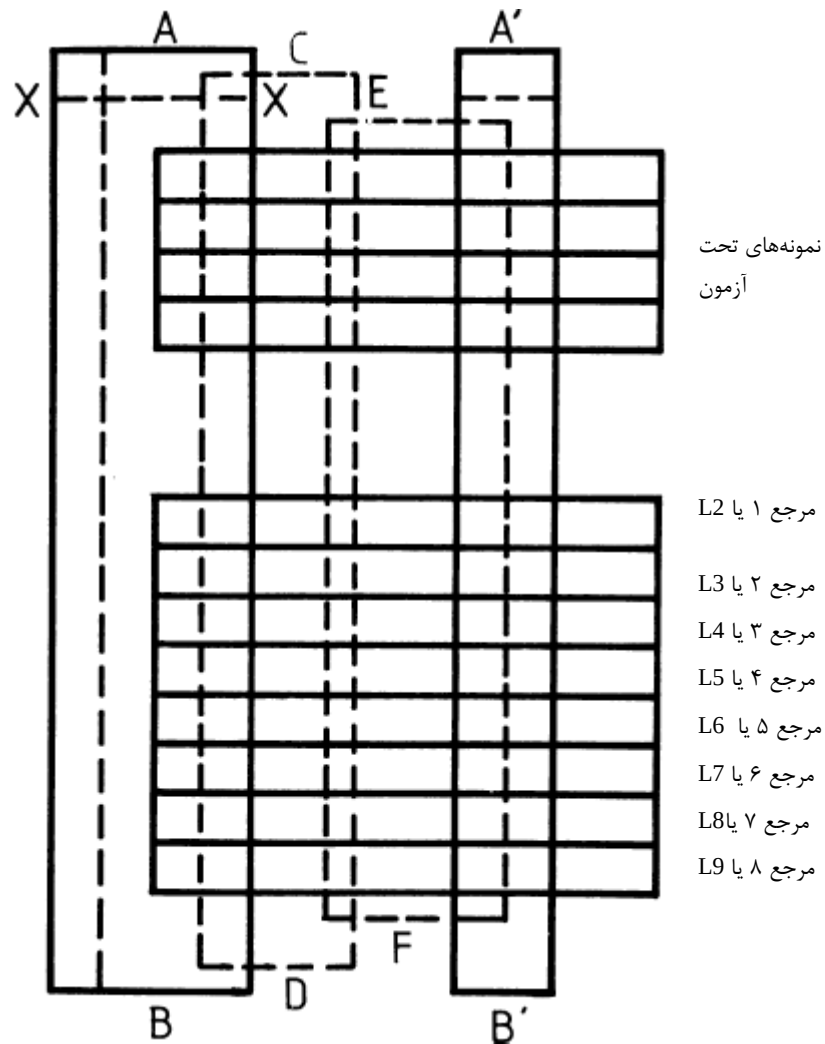
شکل ۳- شمایی از نحوه نصب آزمونه‌ها و مرجع‌ها برای روش ۲
