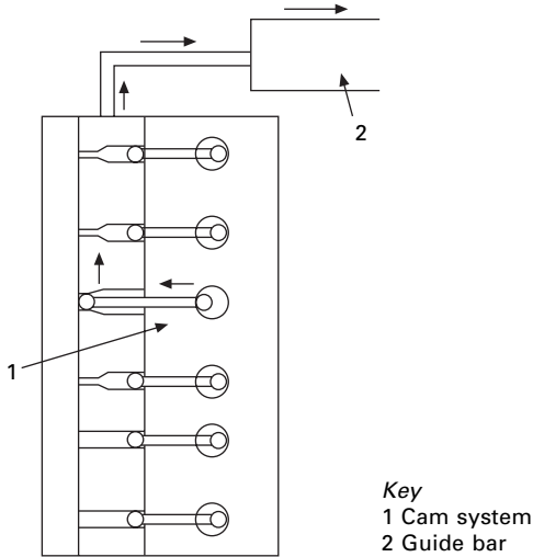
9.58 SU unit.
